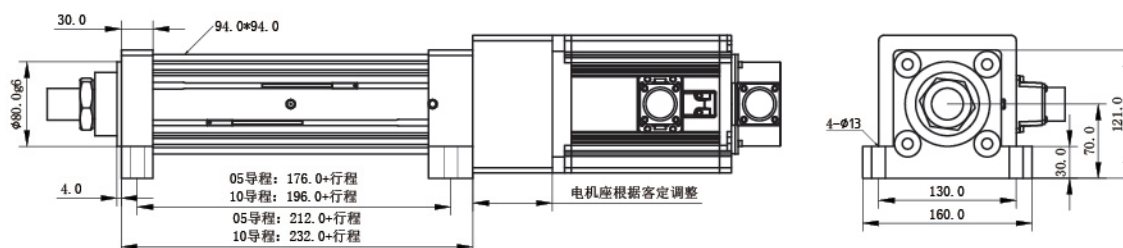
直连式 侧法兰安装
