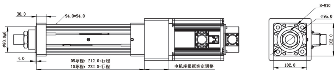
直连式 无法兰安装
