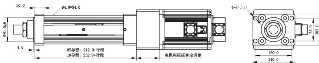
直连式 前法兰安装
